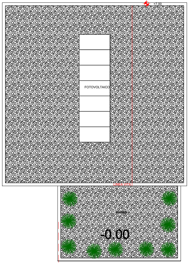
PIANTA COPERTURA
