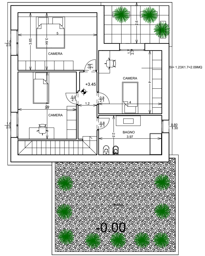
PIANTA PRIMO
