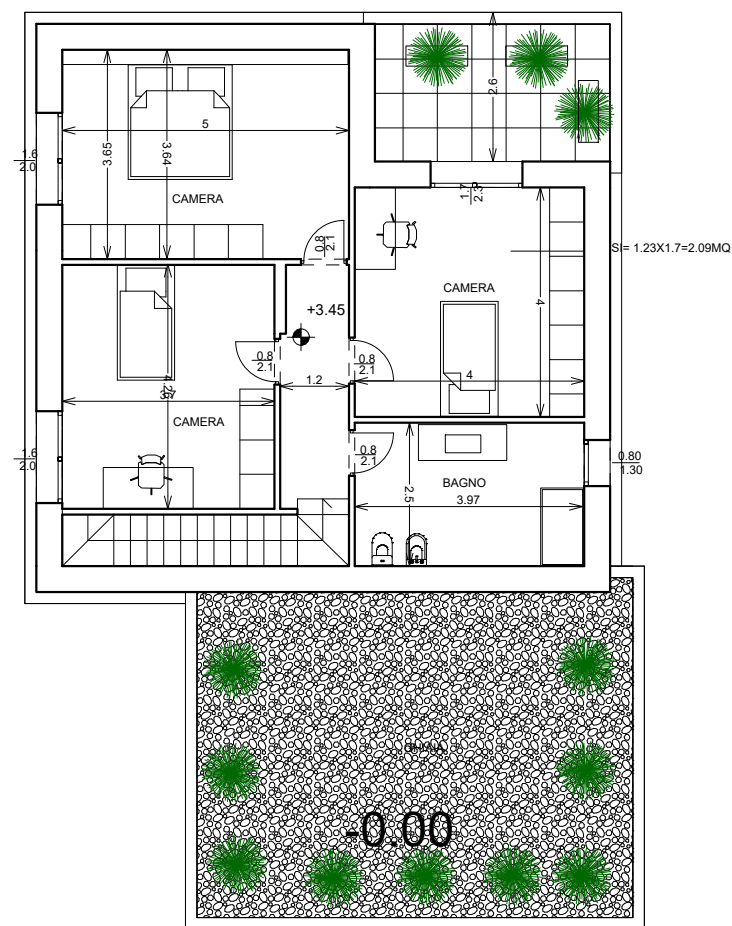
PIANTA PRIMO
