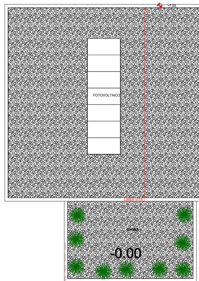
PIANTA COPERTURA
